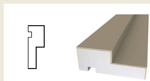
O-32 3 x 8 x 200
